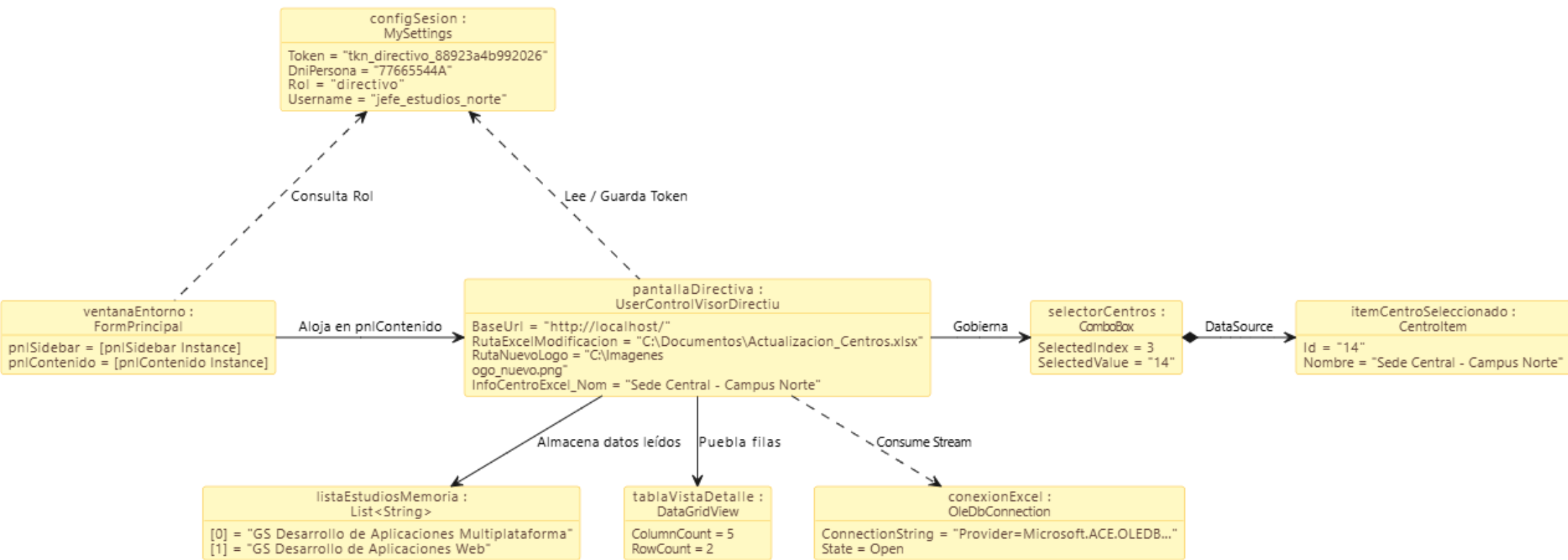
Diagrama de Objetos - Escenario 1: Modificación de Centro (Jefe de Estudios / Directivo)
